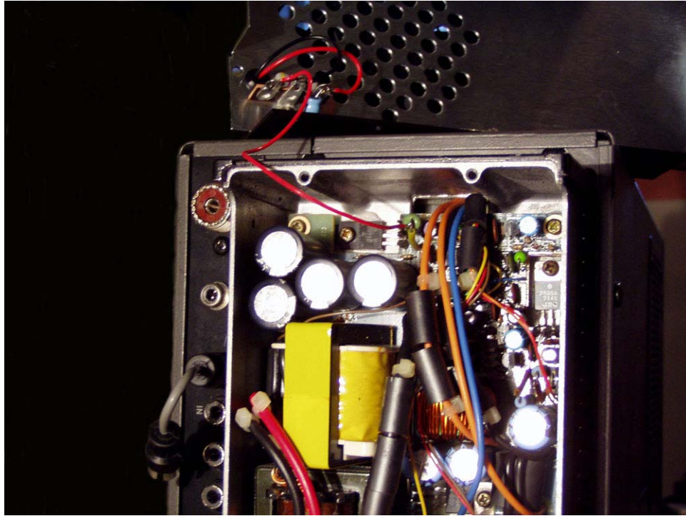
Fan Connections
